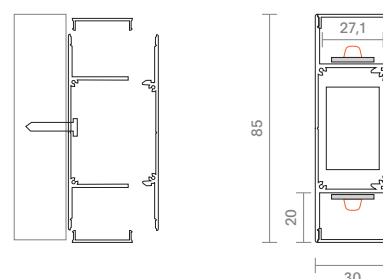
Montageskizze
