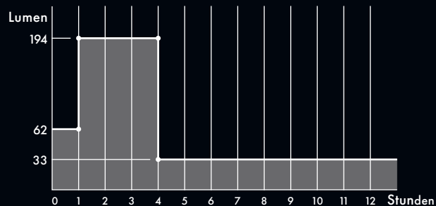
Lumen/Betriebszeit
