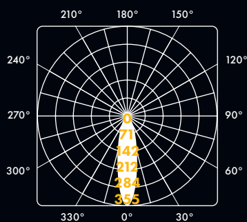
Photometrische Kurve
