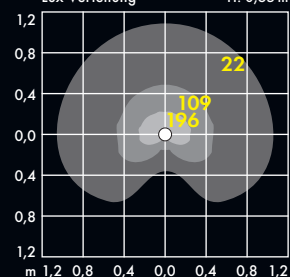
ISO Lux Lux Verteilung STEM MAXI: H: 0,65 m
