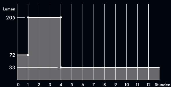
Lumen/Betriebszeit
