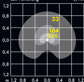
ISO Lux Lux Verteilung STEM MINI: 0,4 m
